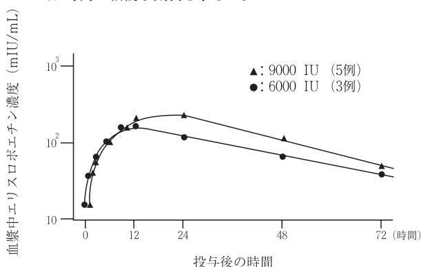
エスポー投与後の血漿中濃度
