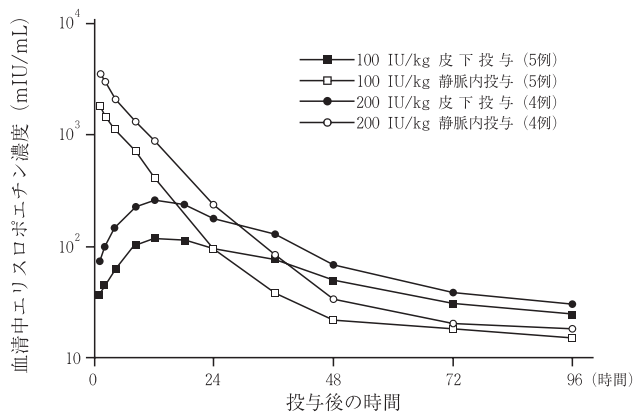
エスポー投与後の血清中濃度推移
